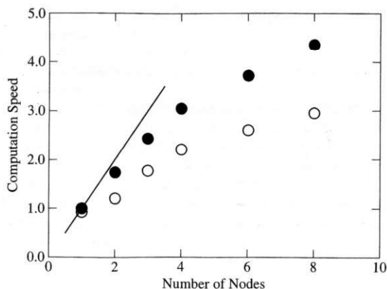
図4 GAMMA 通信 (●) および TCP/IP 通信 (○) 下での、密度汎関数・第一原理分子動力学コード Siesta の正規化された演算速度 (プロセッサ数 1 の能力を 1 とした相対値) とプロセッサ数の関係。測定は Pentium 4 (3.0 GHz), 3Com996 NIC (ギガビットイーサネット), pgf90 v5.1 コンパイラを用いており、直線は正規化された演算速度がプロセッサ数に等しい理想的な場合を表す。演算速度は並列度とともに向上するが、その度合いは GAMMA 通信のほうが TCP/IP 通信よりも大きい。
